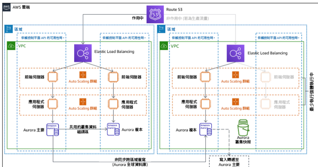
圖 21：暖待命架構
