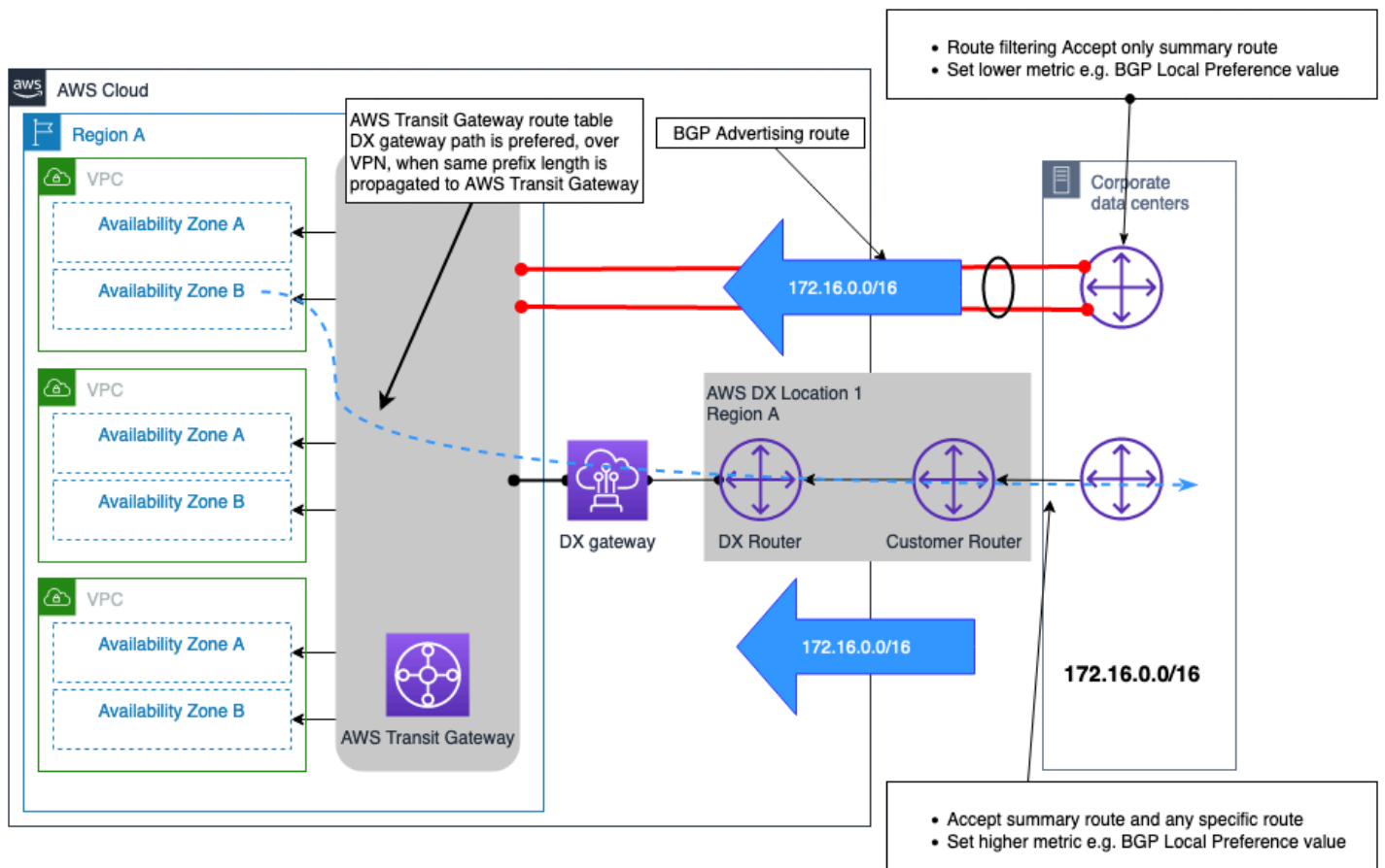
图 12 — VPN 连接作为 AWS DX 的备份连接示例
