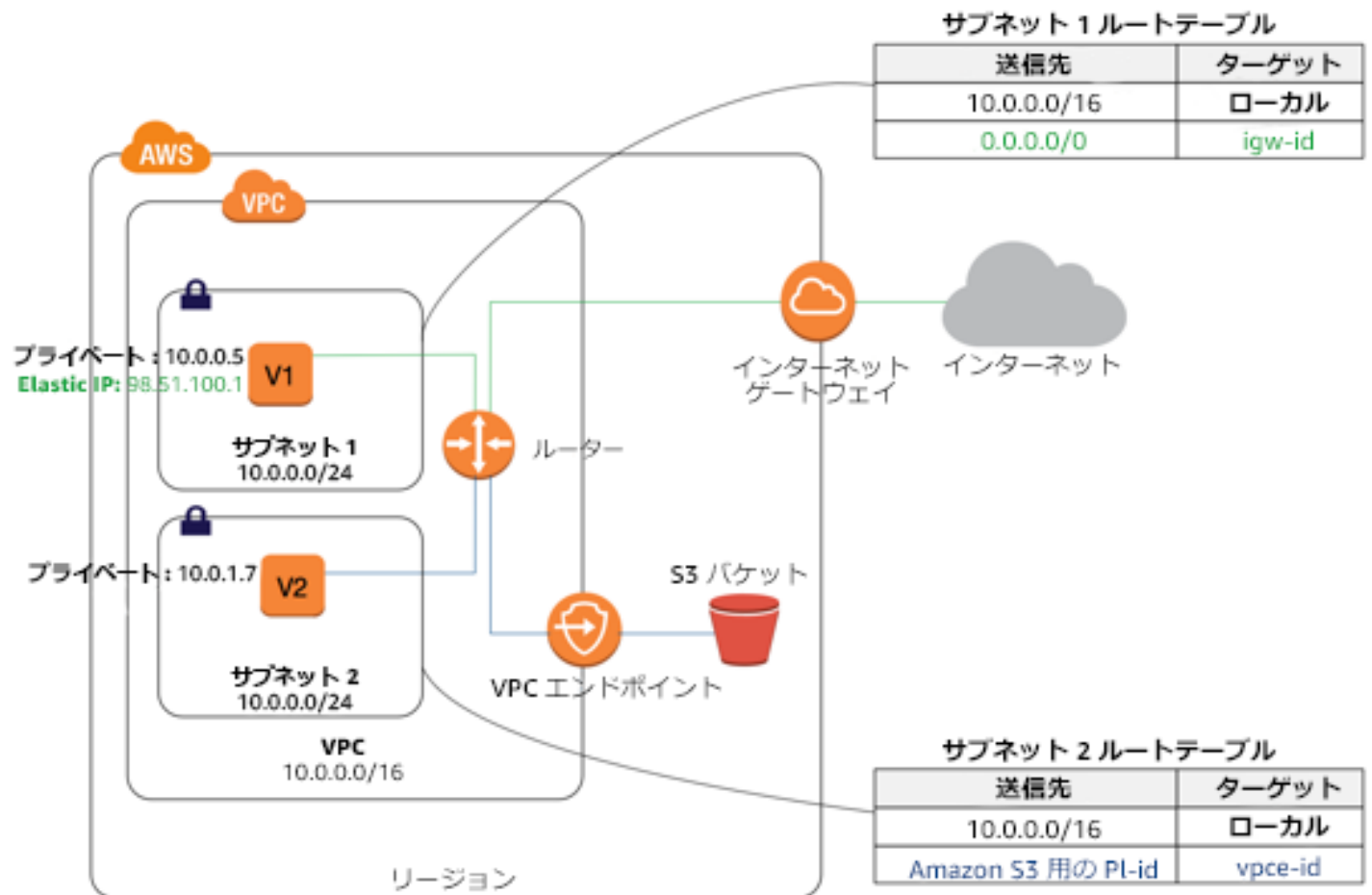
図 7: サブネット 2 のインスタンスは、ゲートウェイエンドポイントを介してのみ Amazon S3 にアクセスできる
