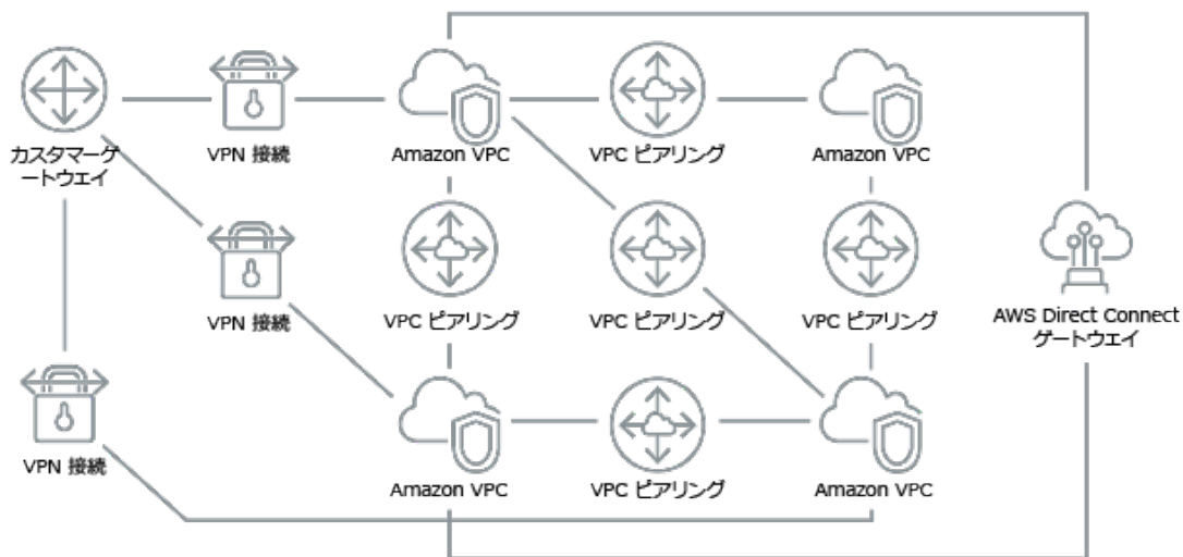
図 1: AWS Transit Gateway なしの場合: VPN 接続を使用して、各 Amazon VPC を相互にピア接続し、オンサイトの各口ケーションをピア接続する必要があります。これは、拡張するにつれ複雑さが増す可能性があります。
