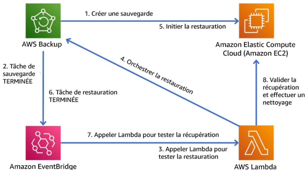
Figure 9 : Processus de sauvegarde et de restauration automatisé
