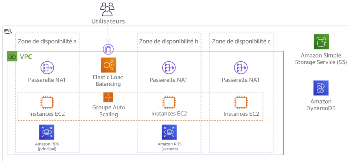
Figure 9 : Architecture multiniveau déployée sur trois zones de disponibilité. Notez qu'Amazon S3 et Amazon DynamoDB comportent toujours automatiquement plusieurs zones de disponibilité. L'ELB est également déployé dans les trois zones.
