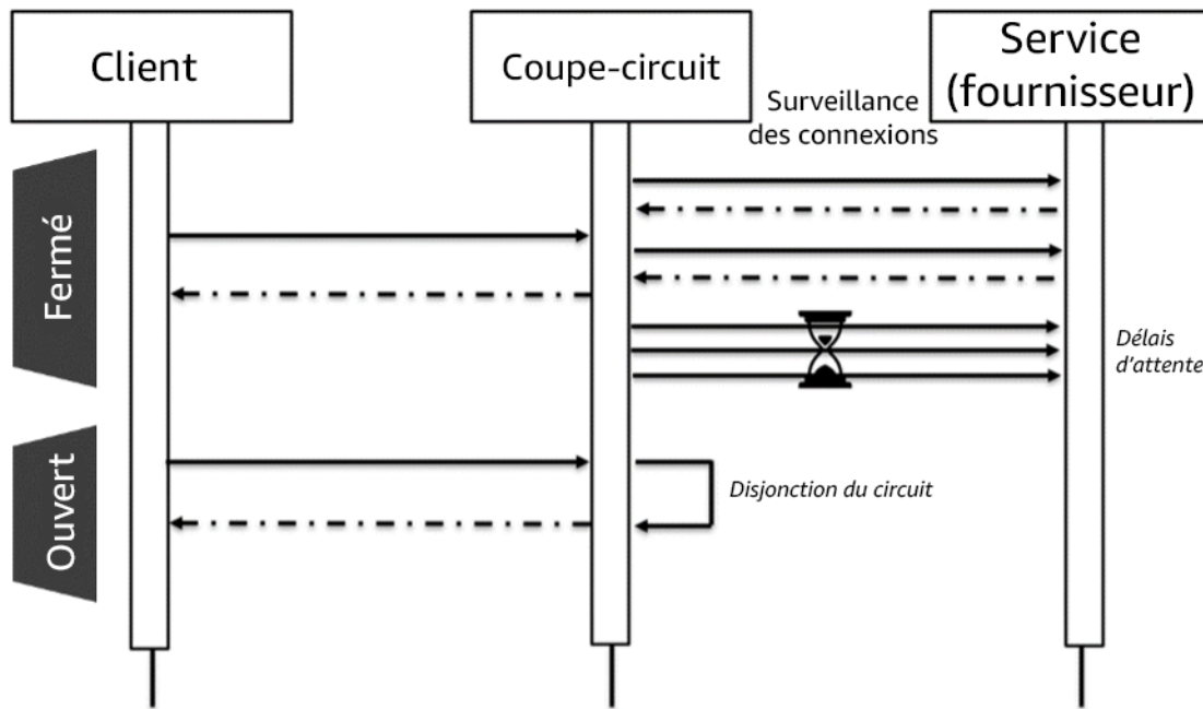
Figure 6 : Coupe-circuit montrant les états fermés et ouverts.
